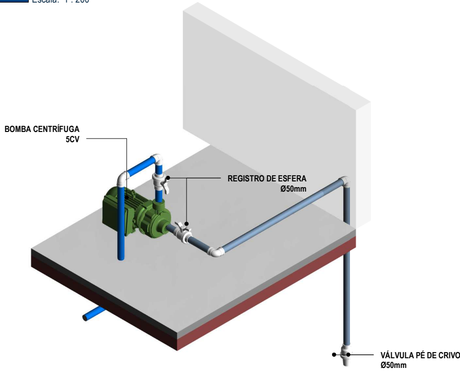
1 2. Térreo Escala: 1: 200
