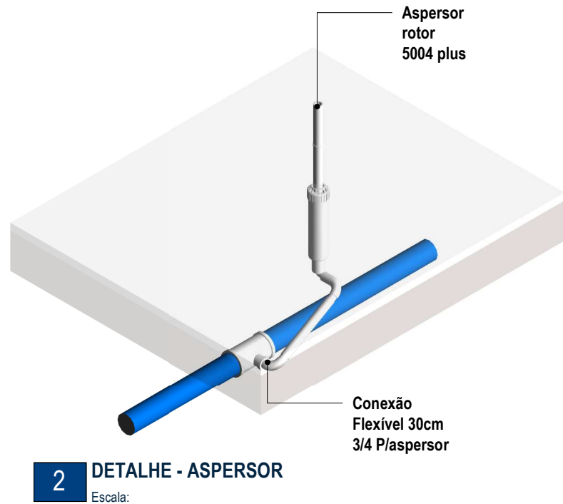
2 DETALHE - ASPERSOR Escala:
